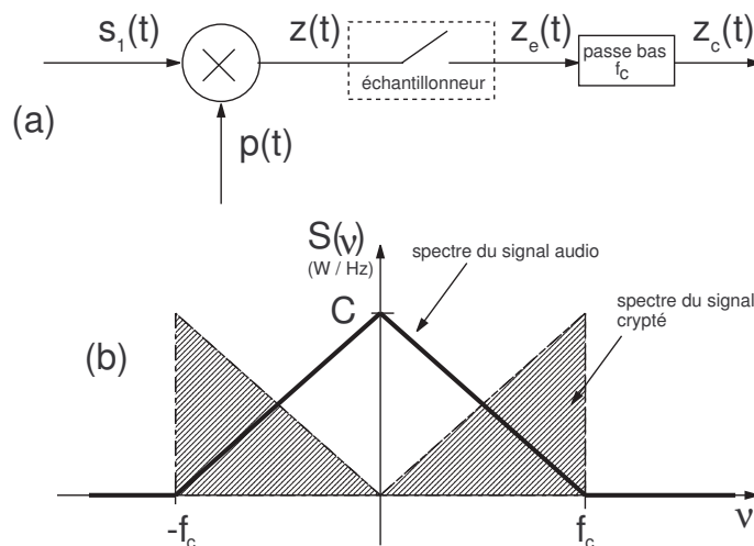
FIGURE 14.55 – (a) : Principe du cryptage d'un signal audio avec un modulateur en anneau. (b) Spectre du signal audio s_1(t) et du signal crypté z_c(t)
