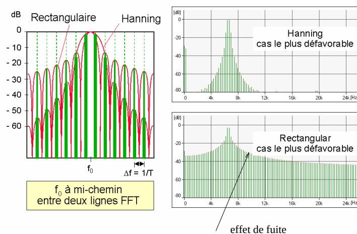
FIGURE 6.10 – La position de la fenêtre de pondération par rapport aux lignes FFT pour engendrer un effet de fuite dans le spectre FFT
