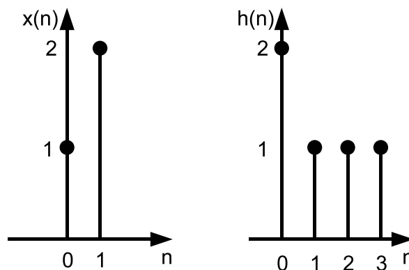
FIGURE 14.111 – Échantillonnage de l'entrée x(t) et de la réponse impulsionnelle h(t) pour le calcul de la convolution numérique y[n]
