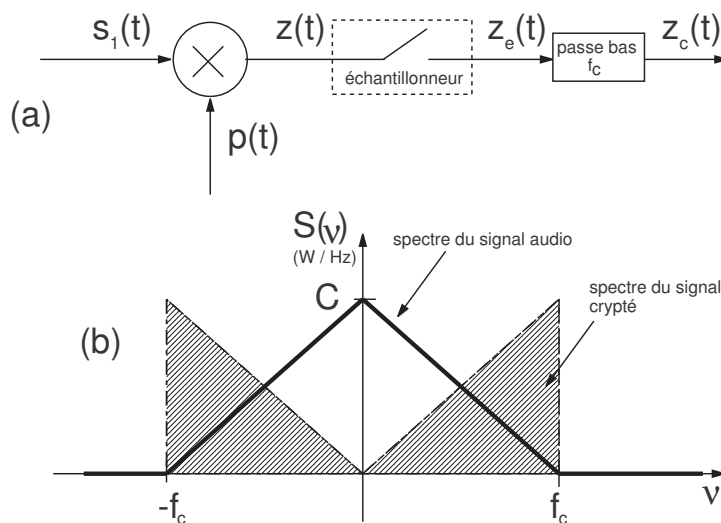
FIGURE 14.118 – (a) : Principe du cryptage d'un signal audio avec un modulateur en anneau. (b) Spectre du signal audio s_1(t) et du signal crypté z_c(t)
