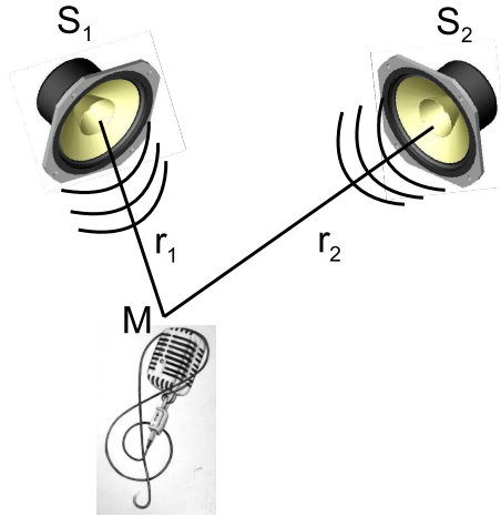
FIGURE 14.110 – Émission stéréophonique d'un signal sonore à partir de deux sources S_1 et S_2
