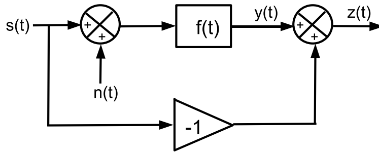
FIGURE 14.122 – Principe schématique du filtrage du signal s(t)
