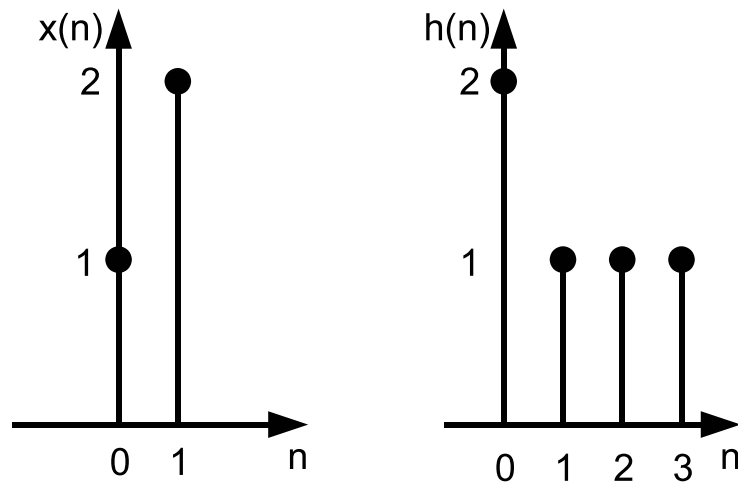
FIGURE 14.87 – Échantillonnage de l'entrée x(t) et de la réponse impulsionnelle h(t) pour le calcul de la convolution numérique y[n]
